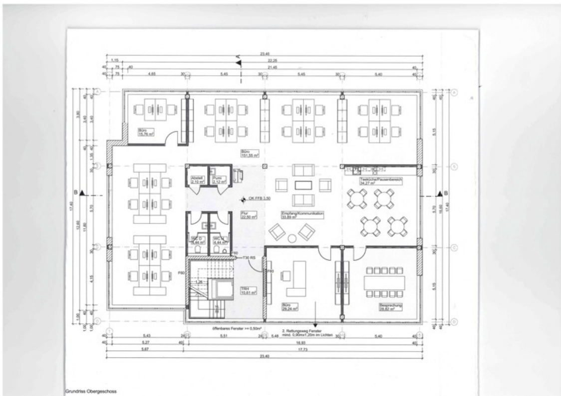
GRUNDRISS
