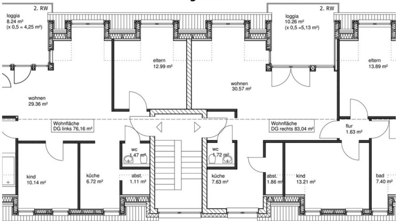
Dachgeschoss
