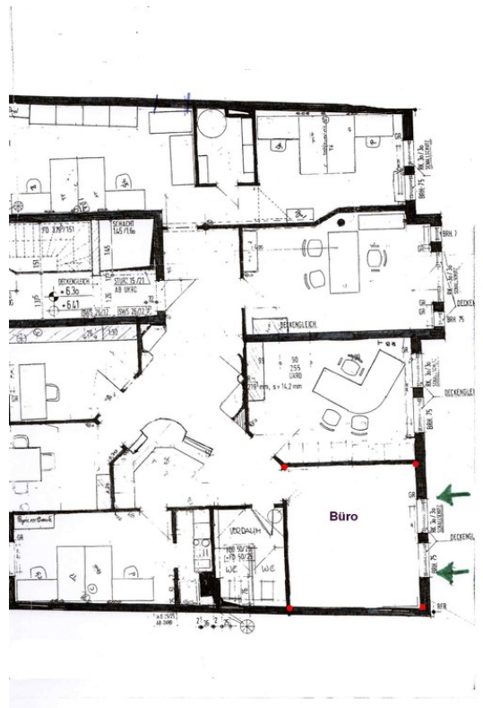
Grundriss Büro
