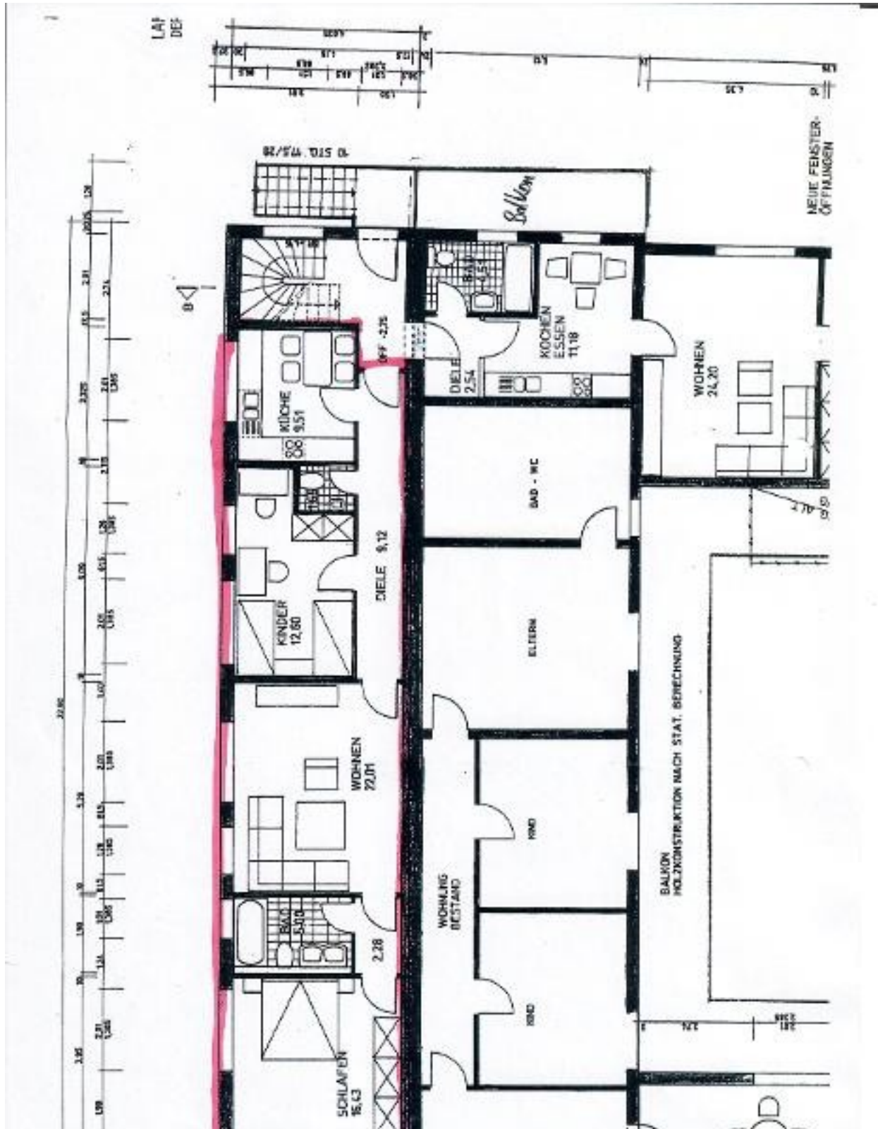
Grundriss EG
