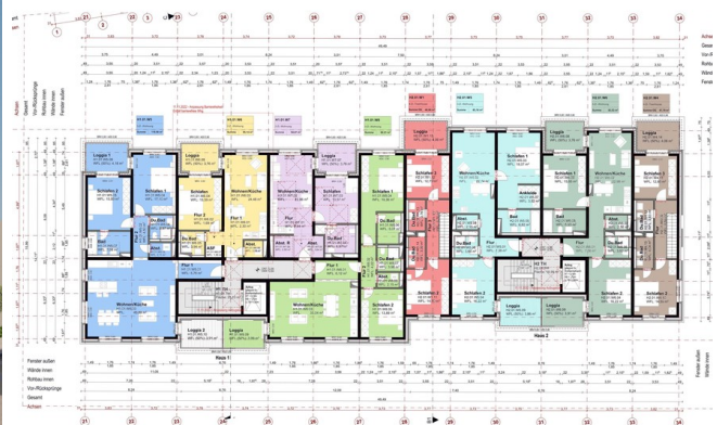
Grundriss 1.Obergeschoss
