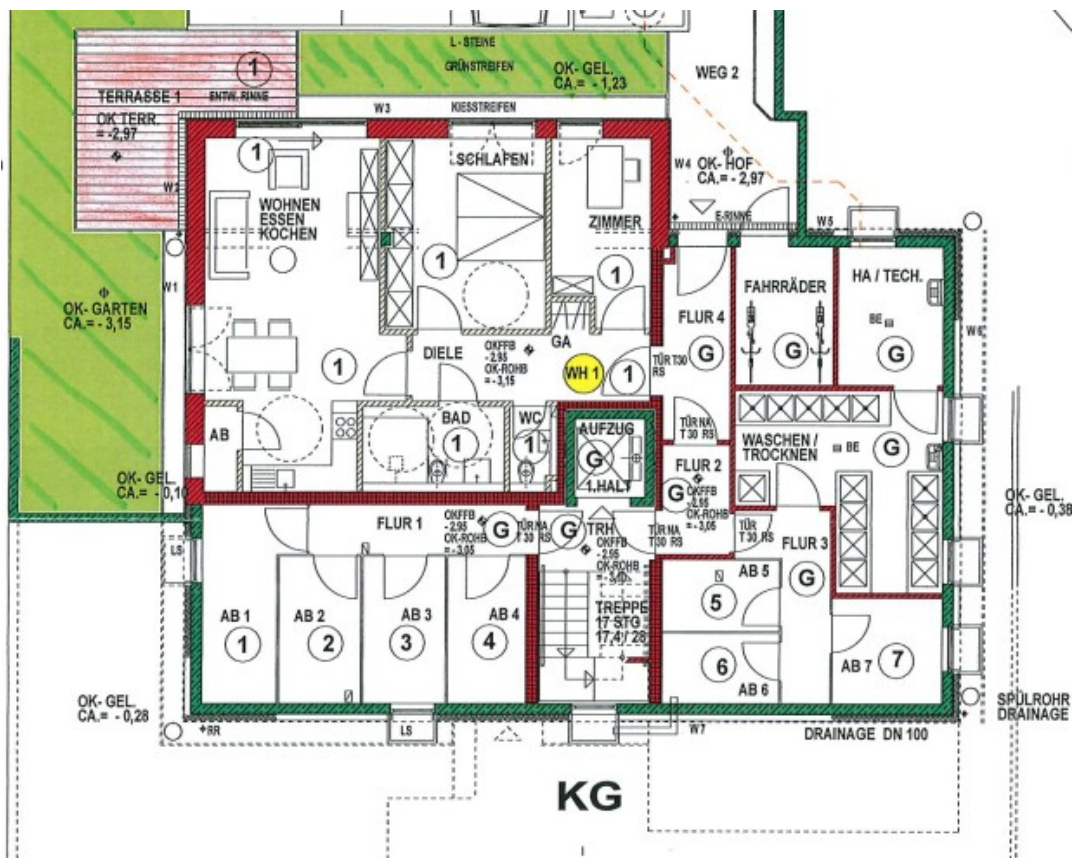
Untergeschoss
