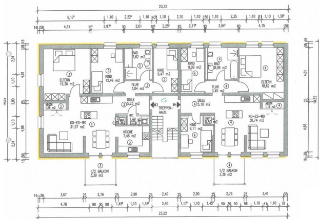
1. Obergeschoss
