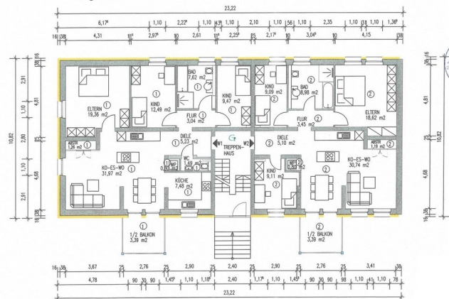
Erdgeschoss
