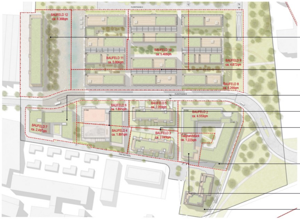
Lageplan | Übersicht Baufelder
