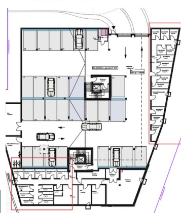
Übersichtsplan Tiefgarage | Keller
