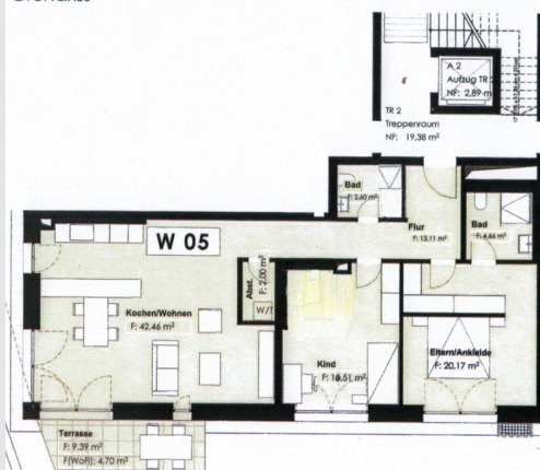
Grundriss
