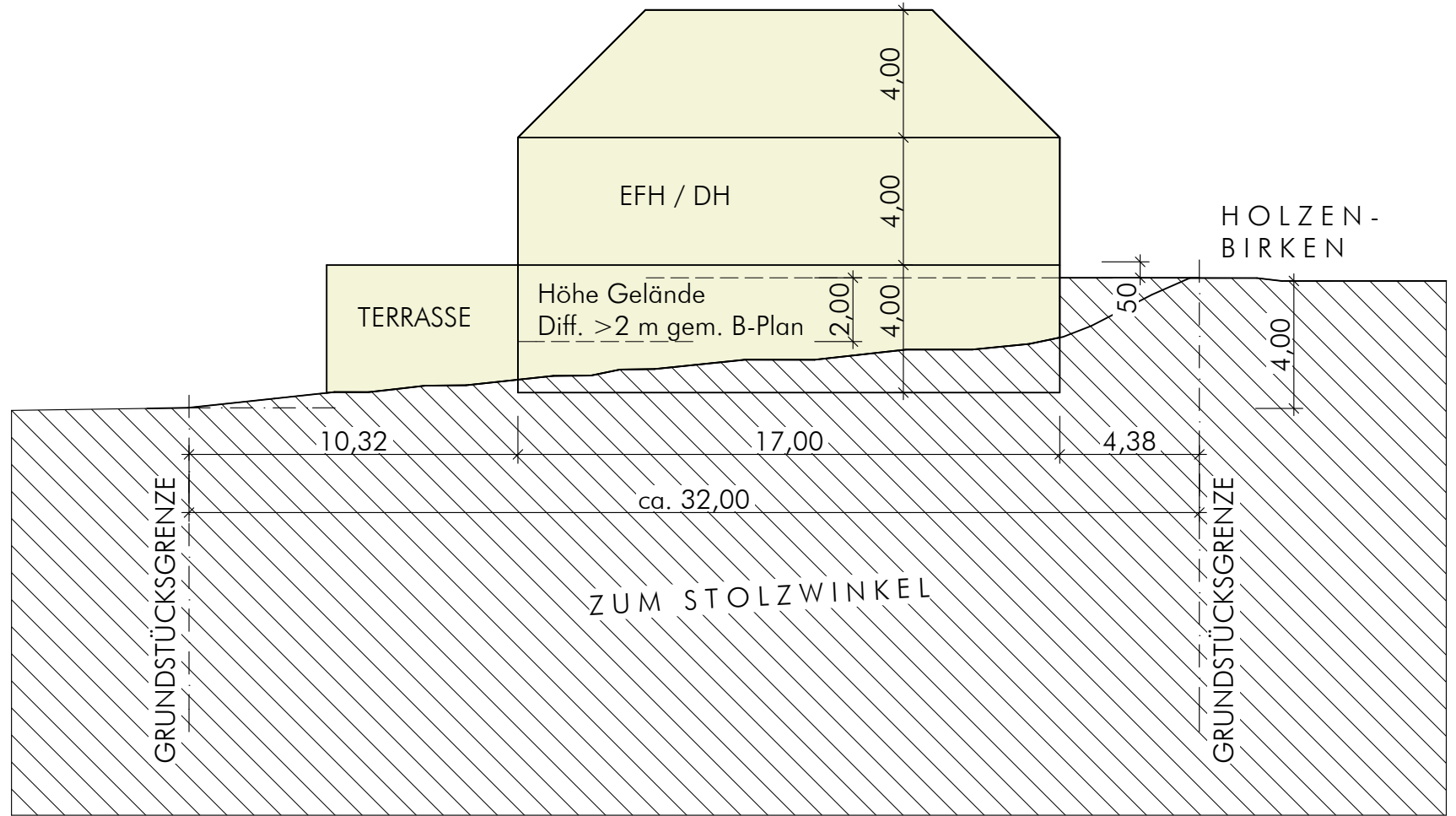
SCHNITT GELÄNDE A-A LAGEPLAN M.1:200
