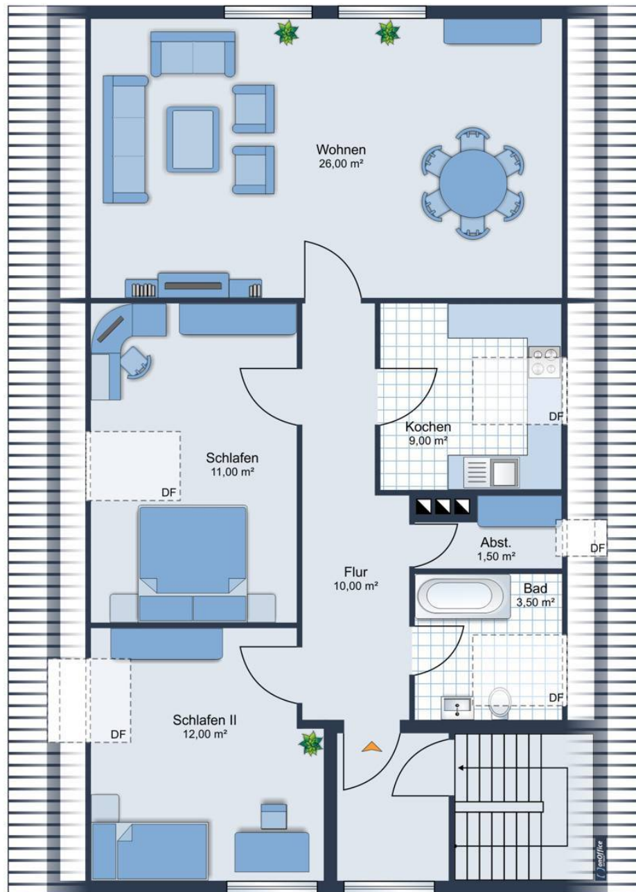
GRUNDRISS
