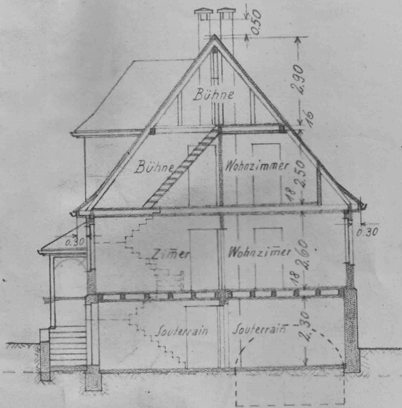
Schnitt A-B.
