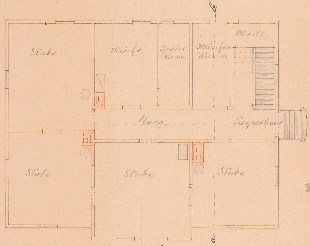
Grundriß Maasstab 1:100
