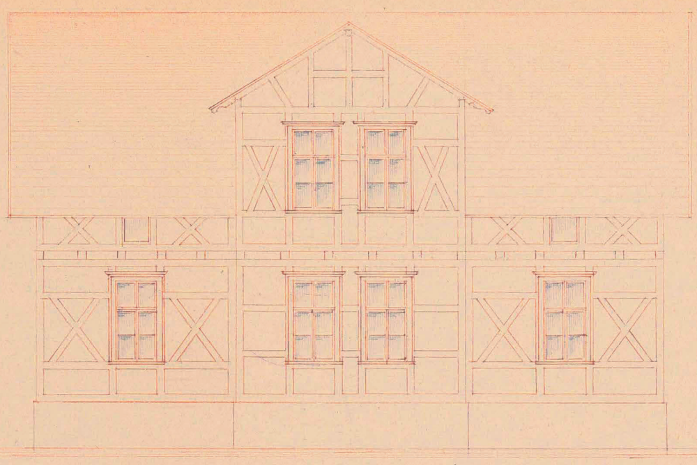
Vorder-Ansicht
