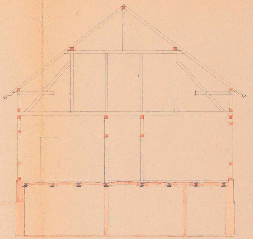
Querschnitt a-b.
