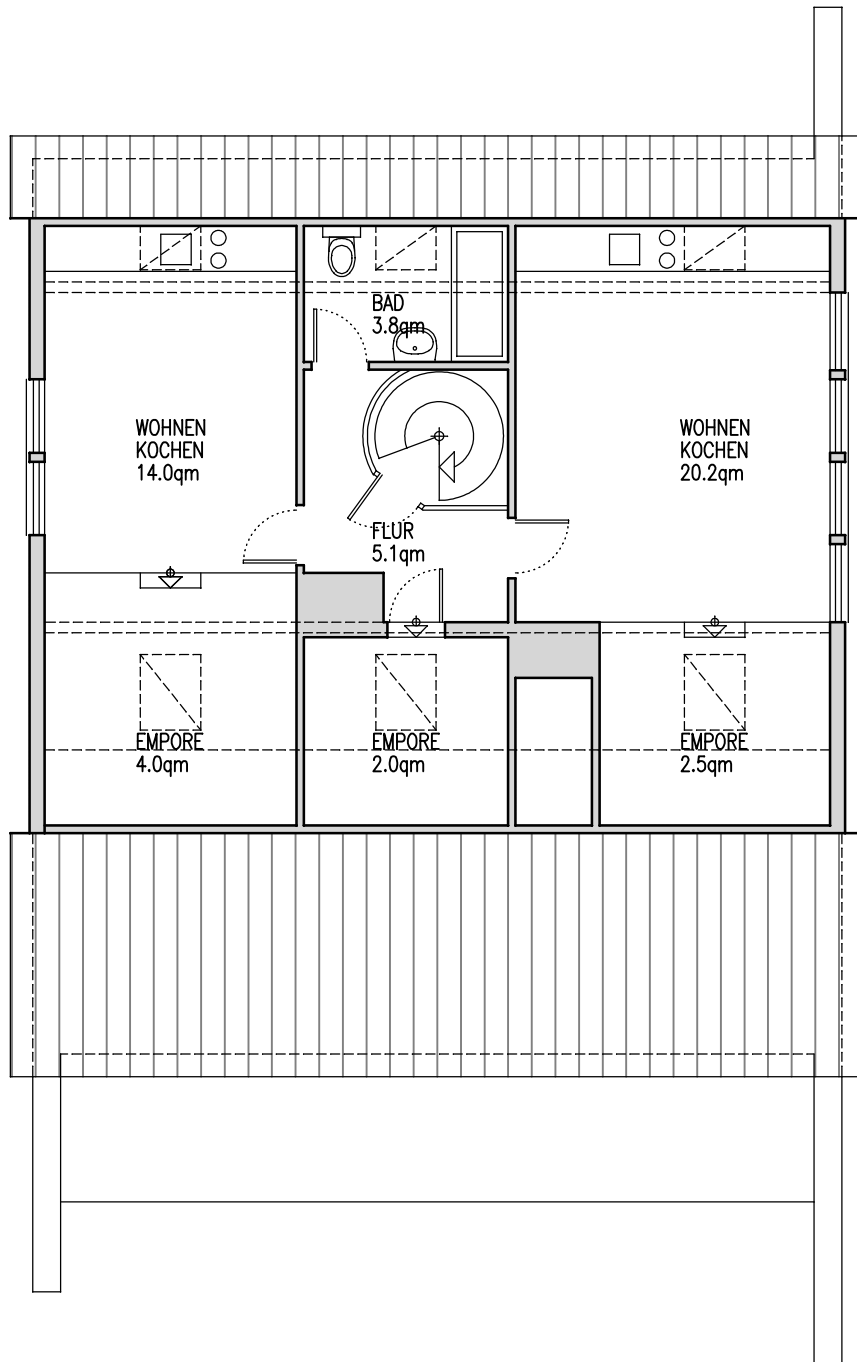
DACHGESCHOSS
