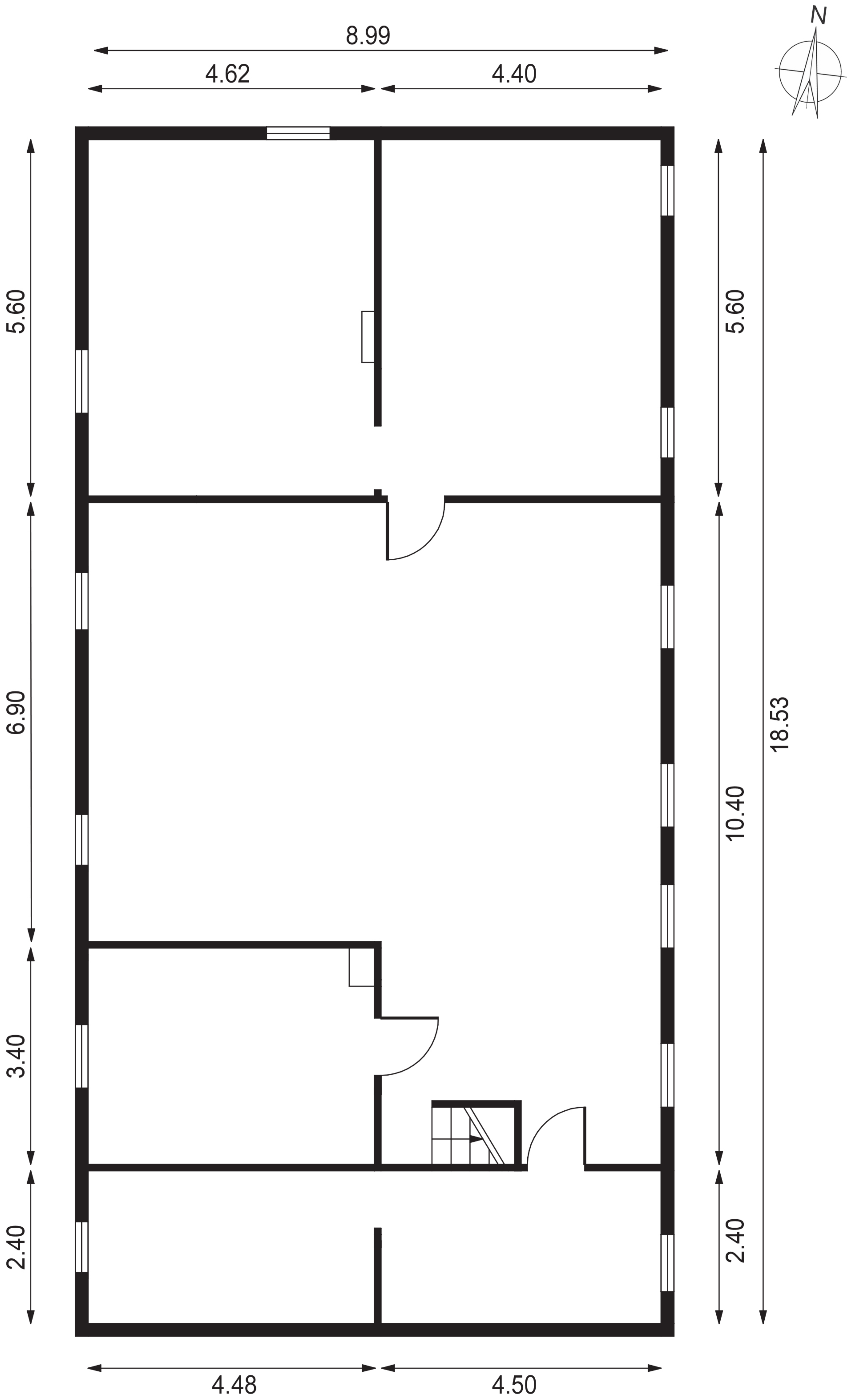
Dachgeschoss
