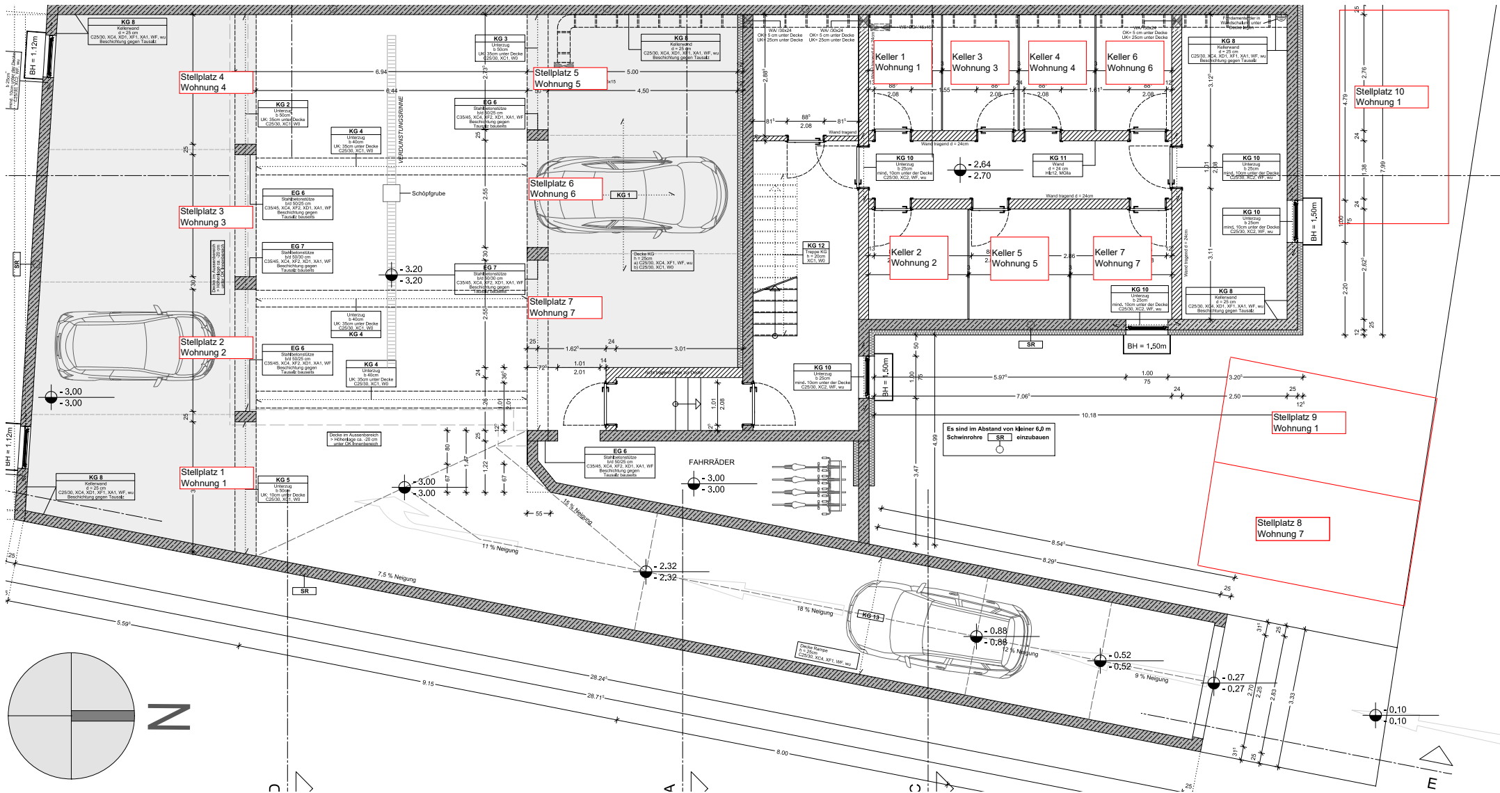
Garagen- und Stellplatzübersicht M 1:125 (Rohbaumaße, tatsächliche Abmessungen können abweichen)
