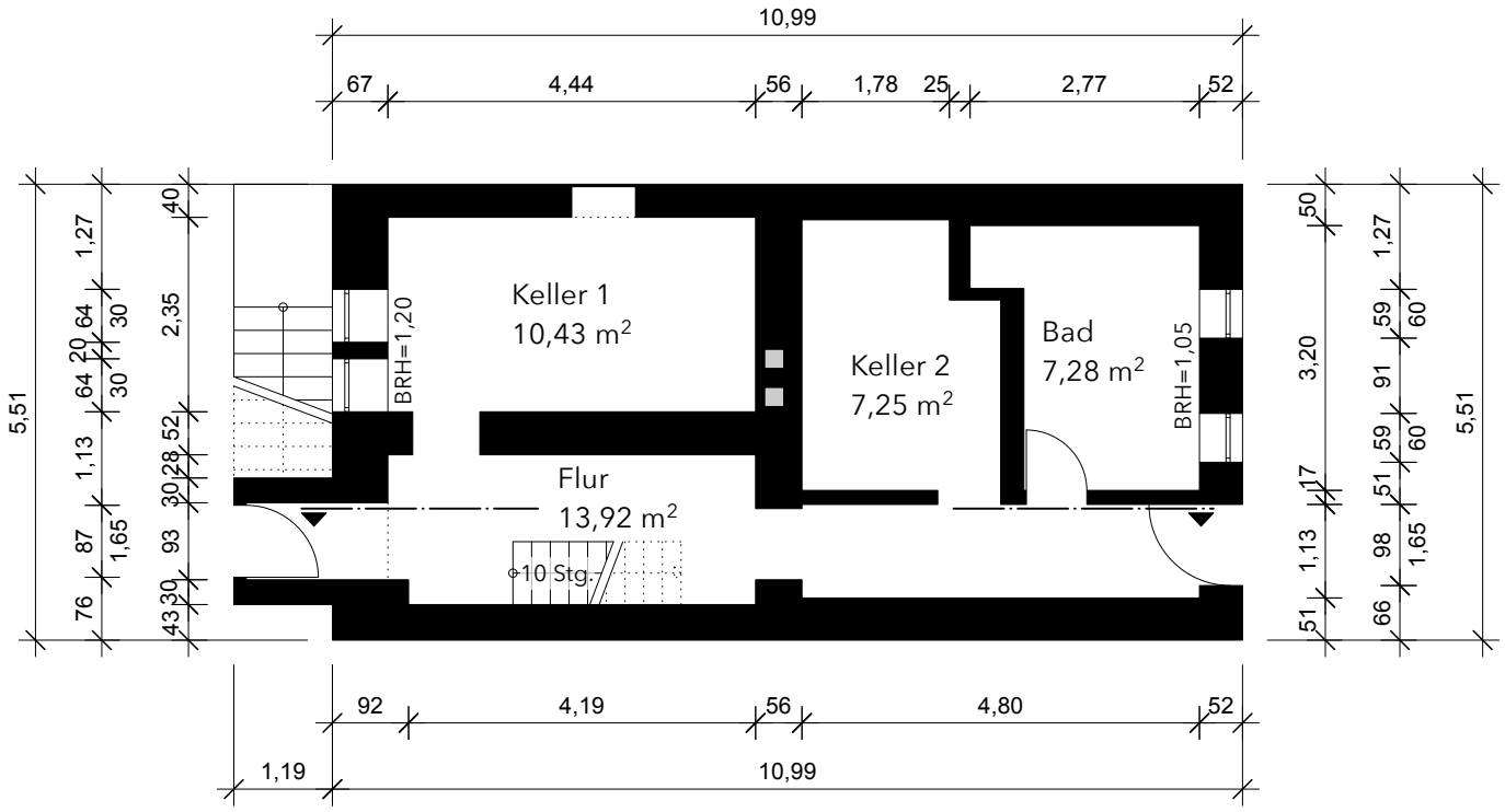
Grundriss KG
