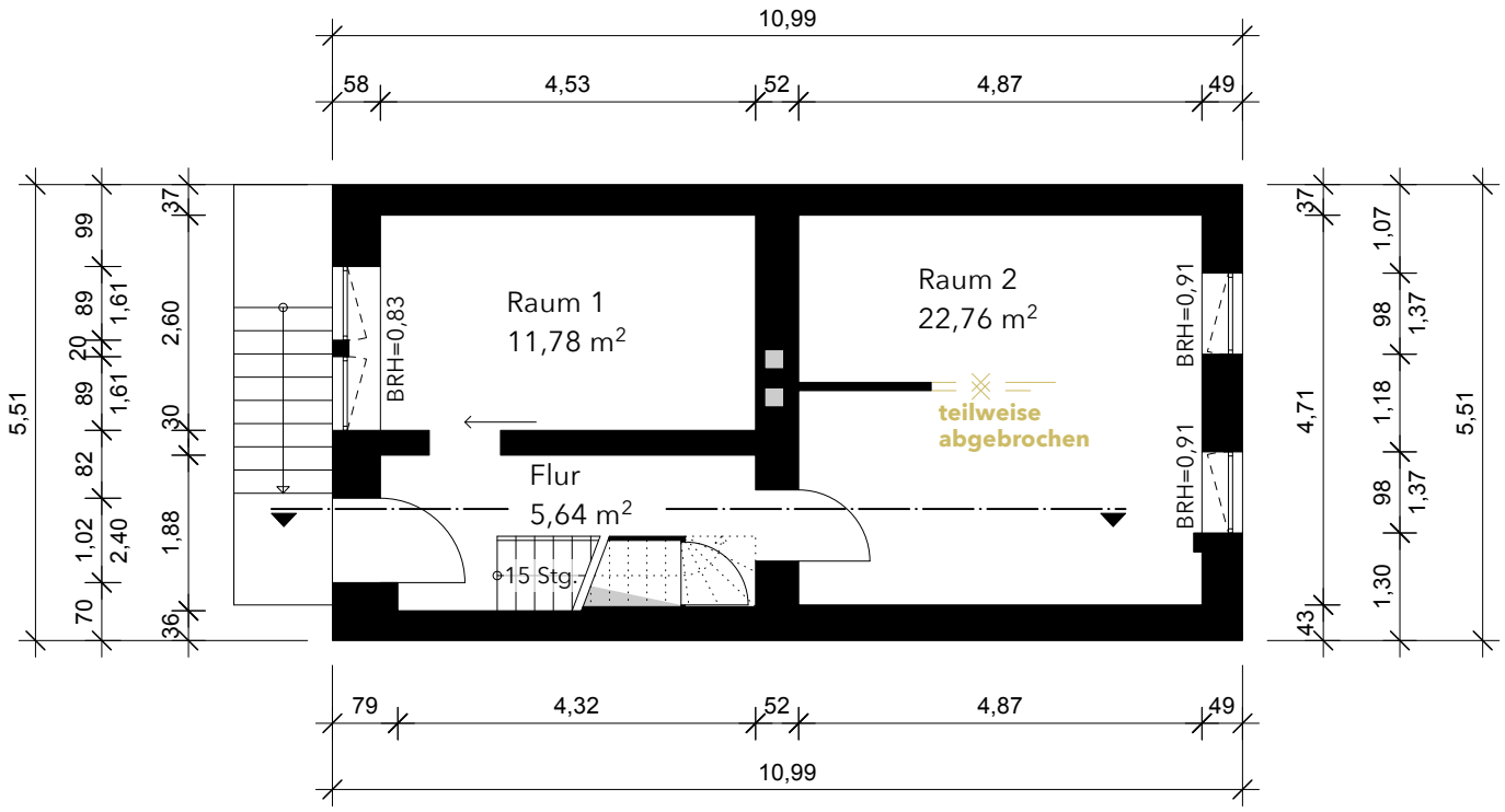
Grundriss EG
