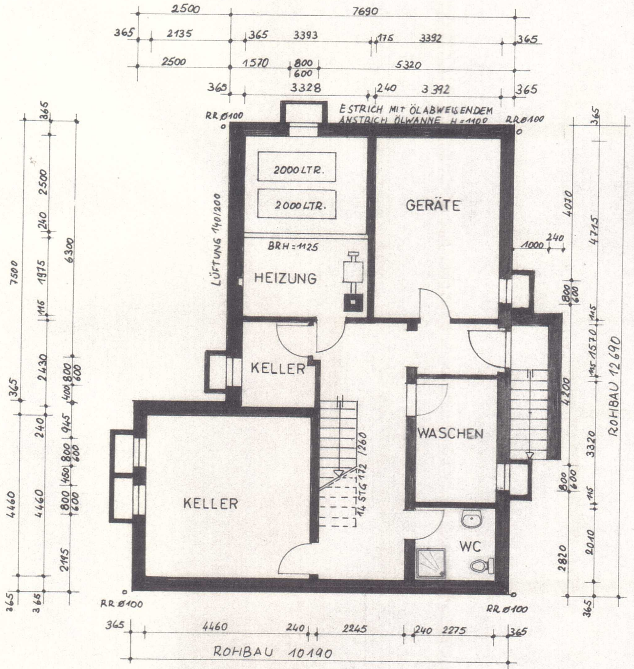
KELLERGRUNDRISS (DECKBLATT)
