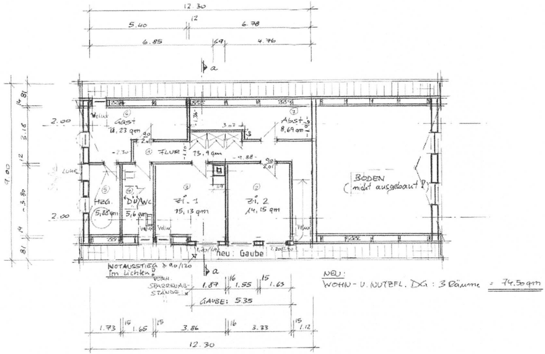
Ausbau Dachgeschoss Grundriss 2010
