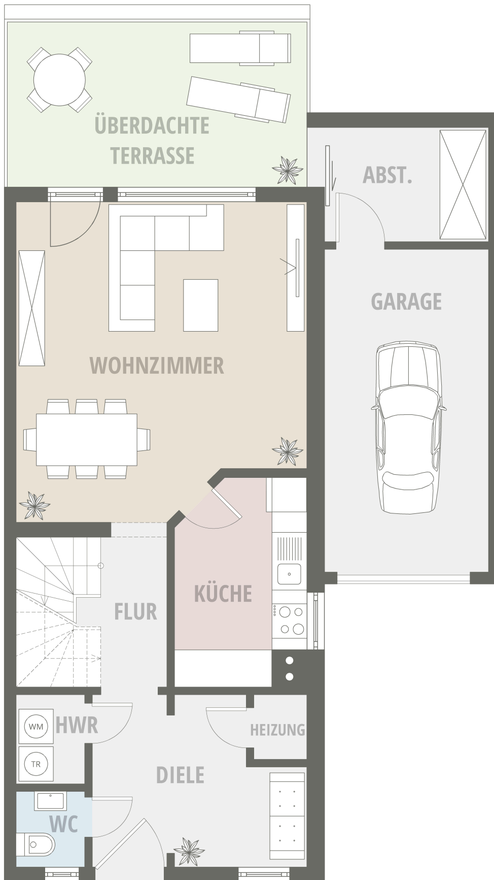
Erdgeschoss
