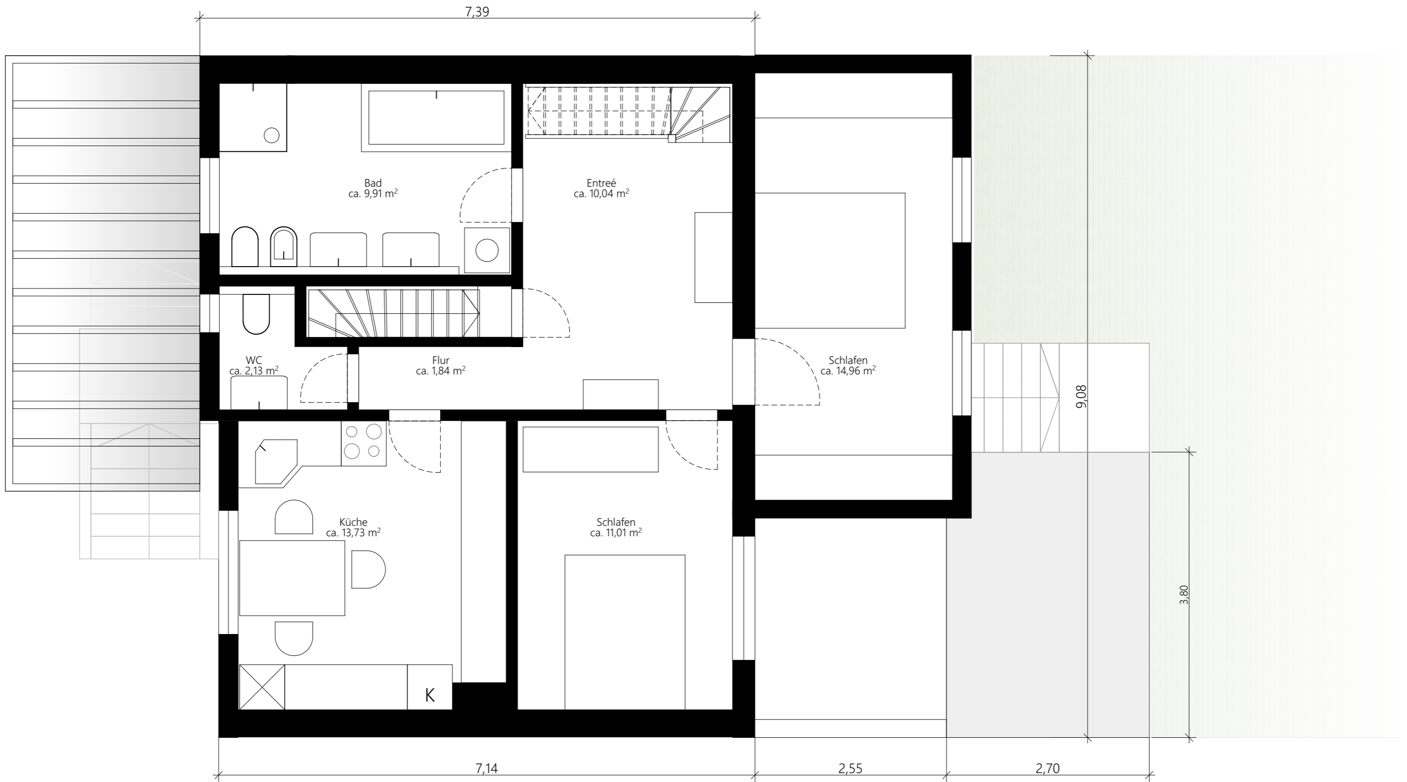
1. Obergeschoss
