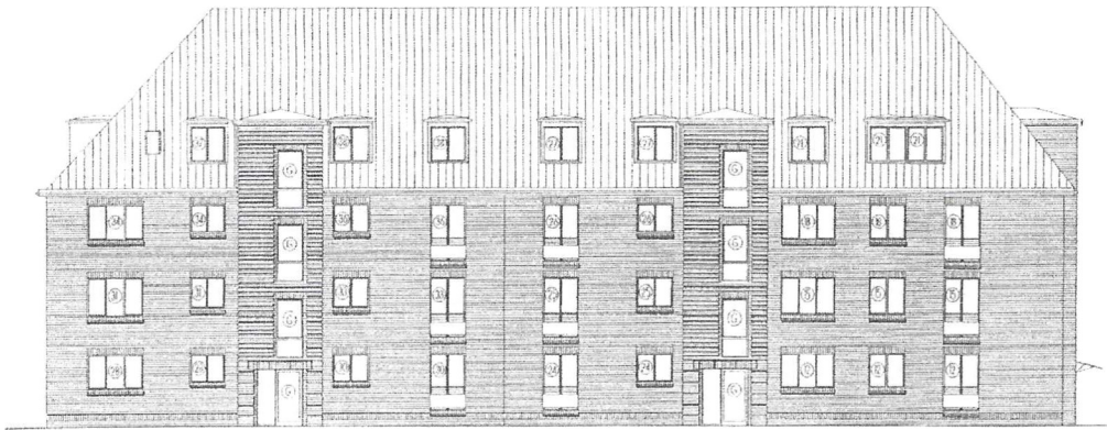
Nordansicht
