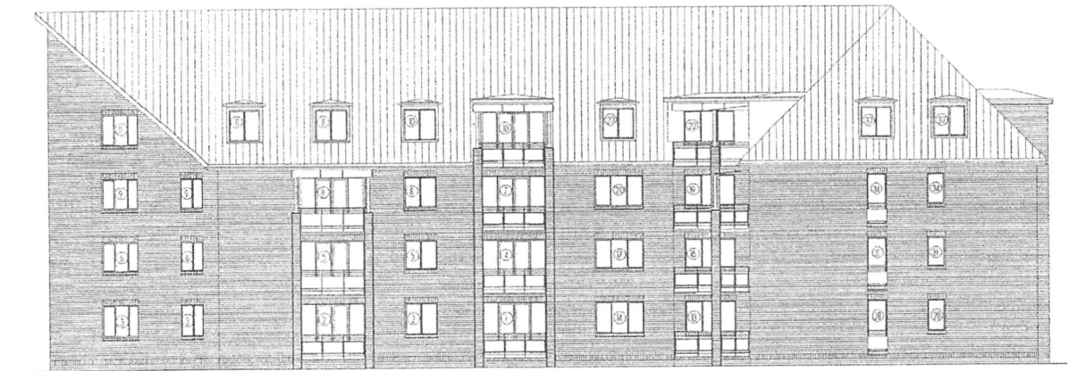
Ostansicht
