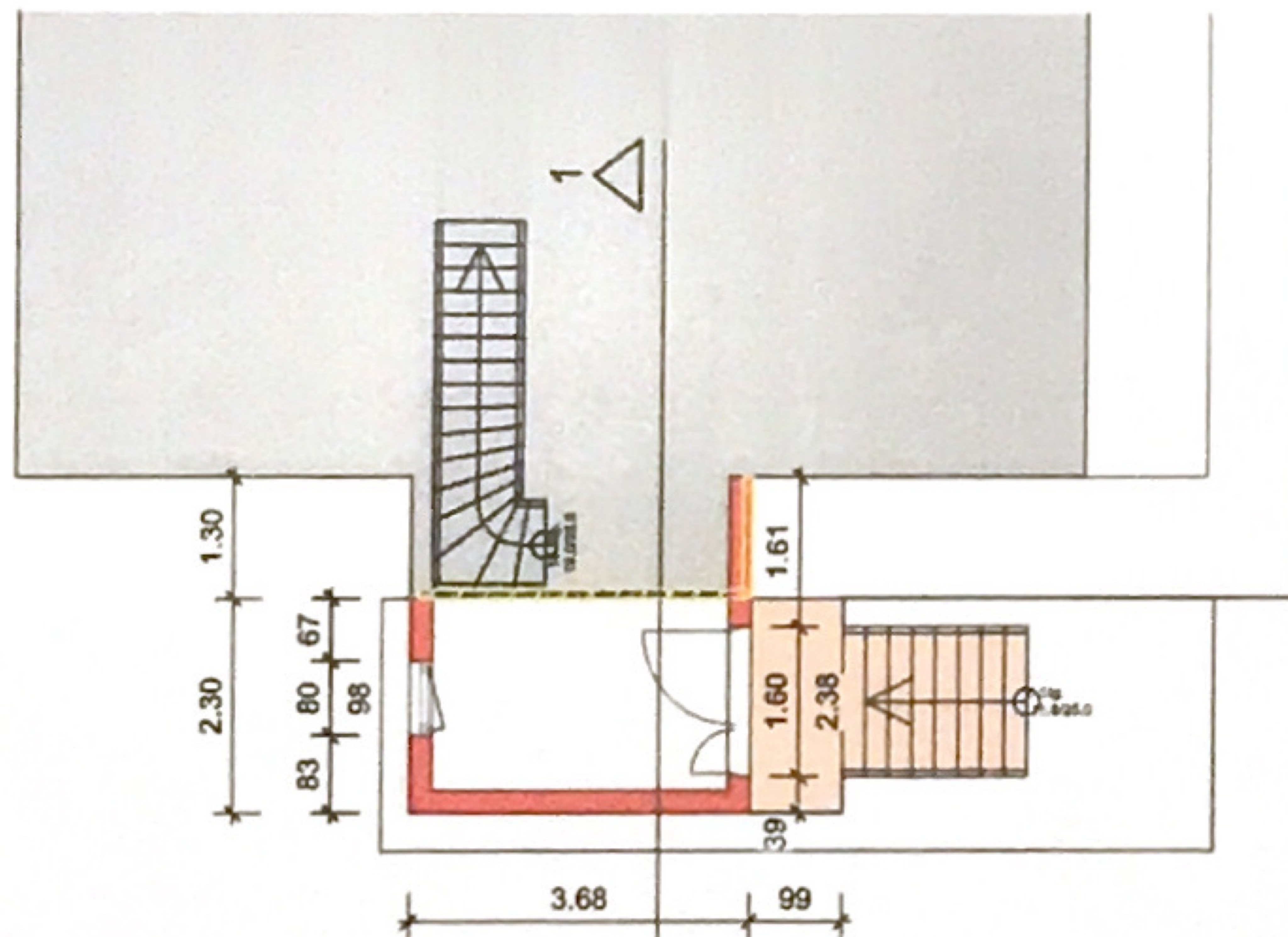
EG M 1 : 100
