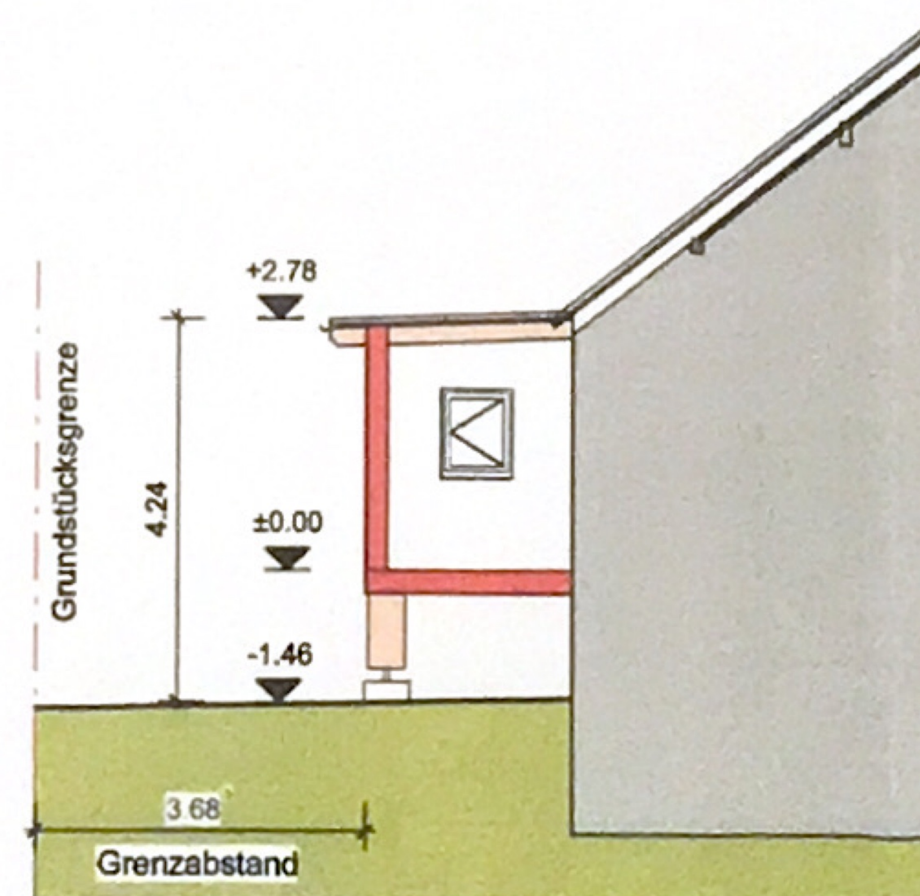
Schnitt 1 - 1 M 1 : 100
