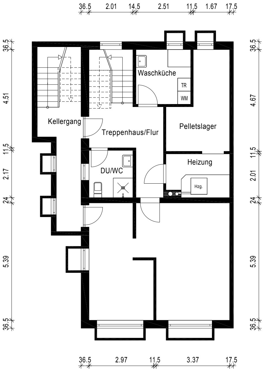
Kellergeschoss
