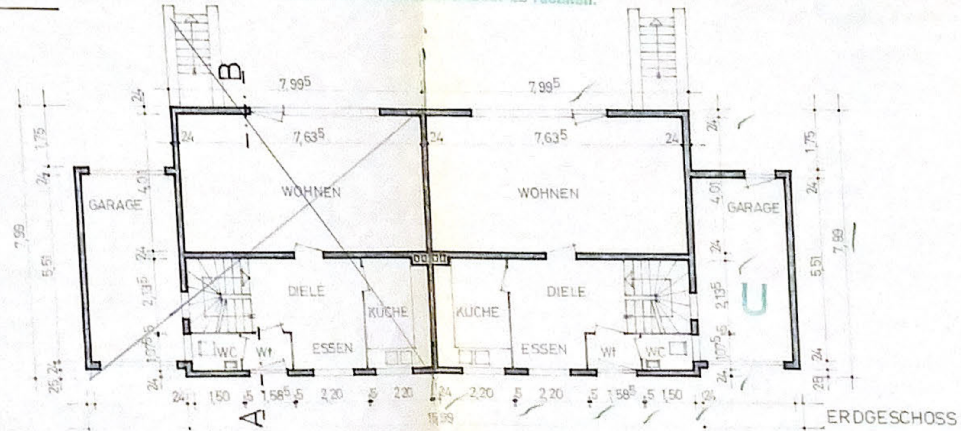
KELLERGESCHOSS
