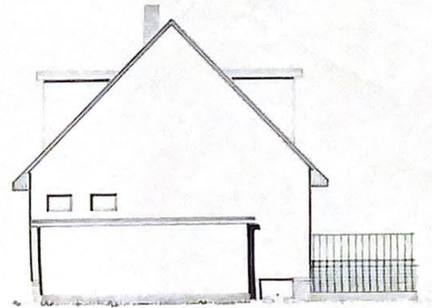
SEITENANSICHT (SÜD)
