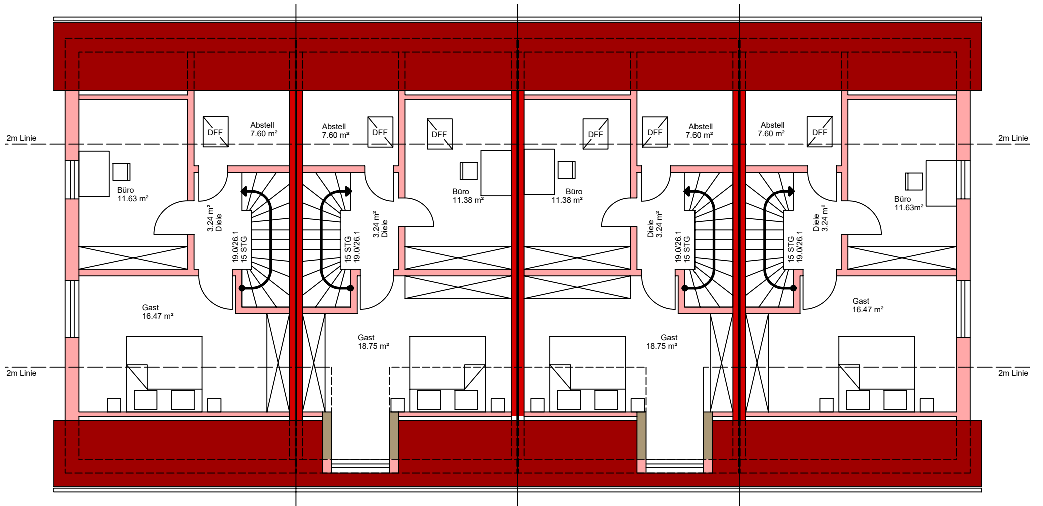
Dachgeschoss
