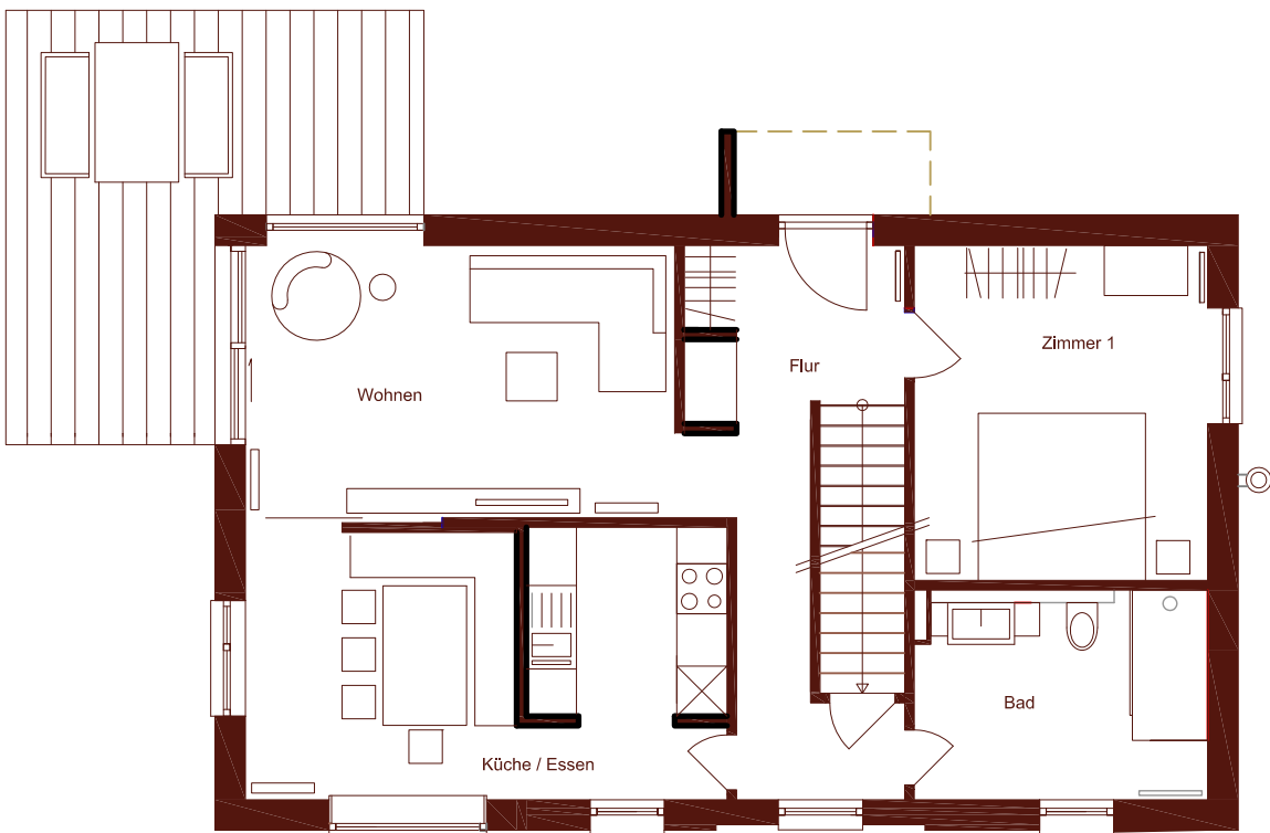
Erdgeschoss
