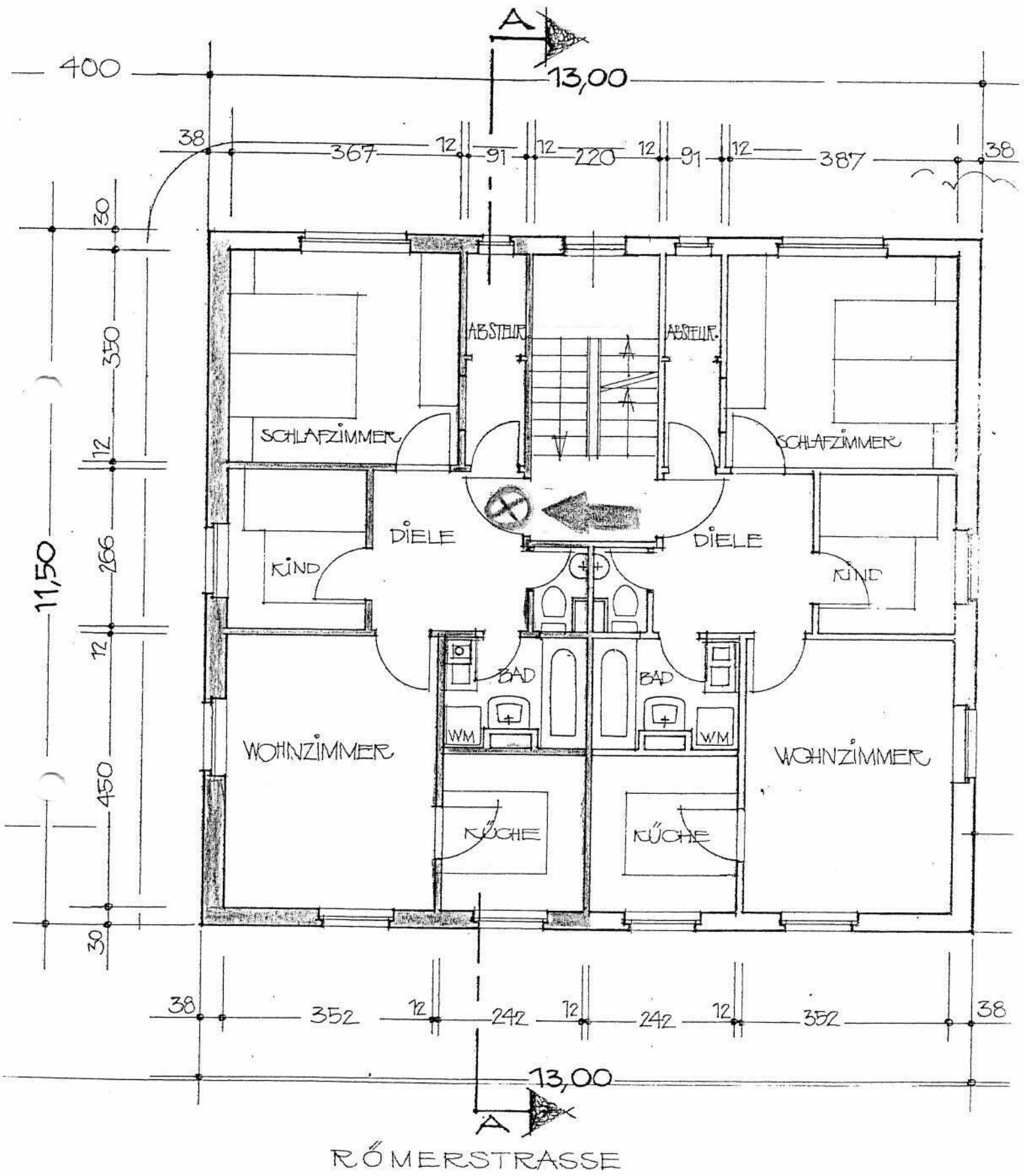
1. OBERGESCHOSS
