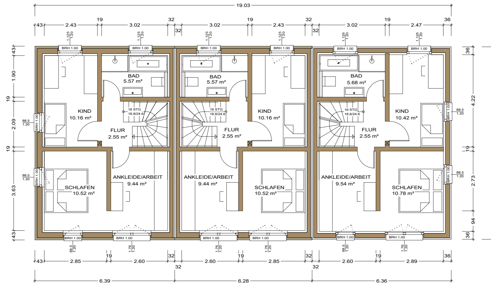
GRUNDRISS OBERGESCHOSS
