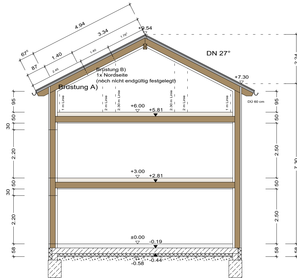
SYSTEMSCHNITT
