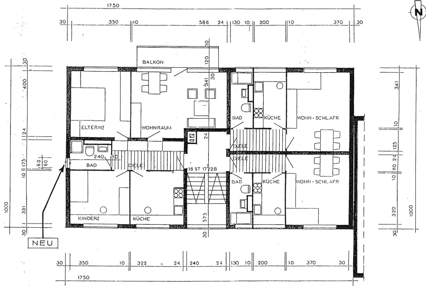
GRUNDRISS ERD.- 1. und 2. OBERGESCHOSS
