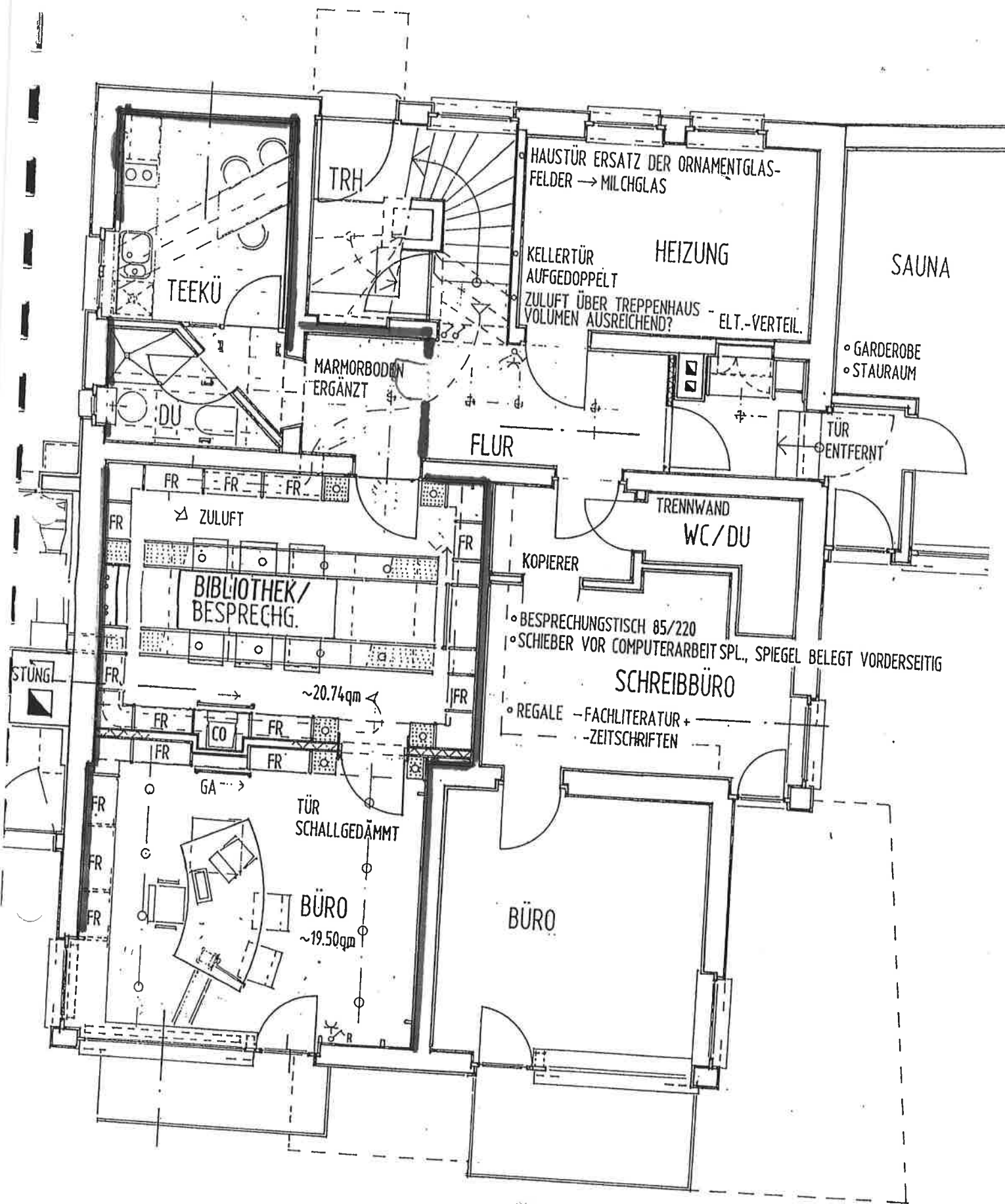
GRUNDRISS 1.UG
