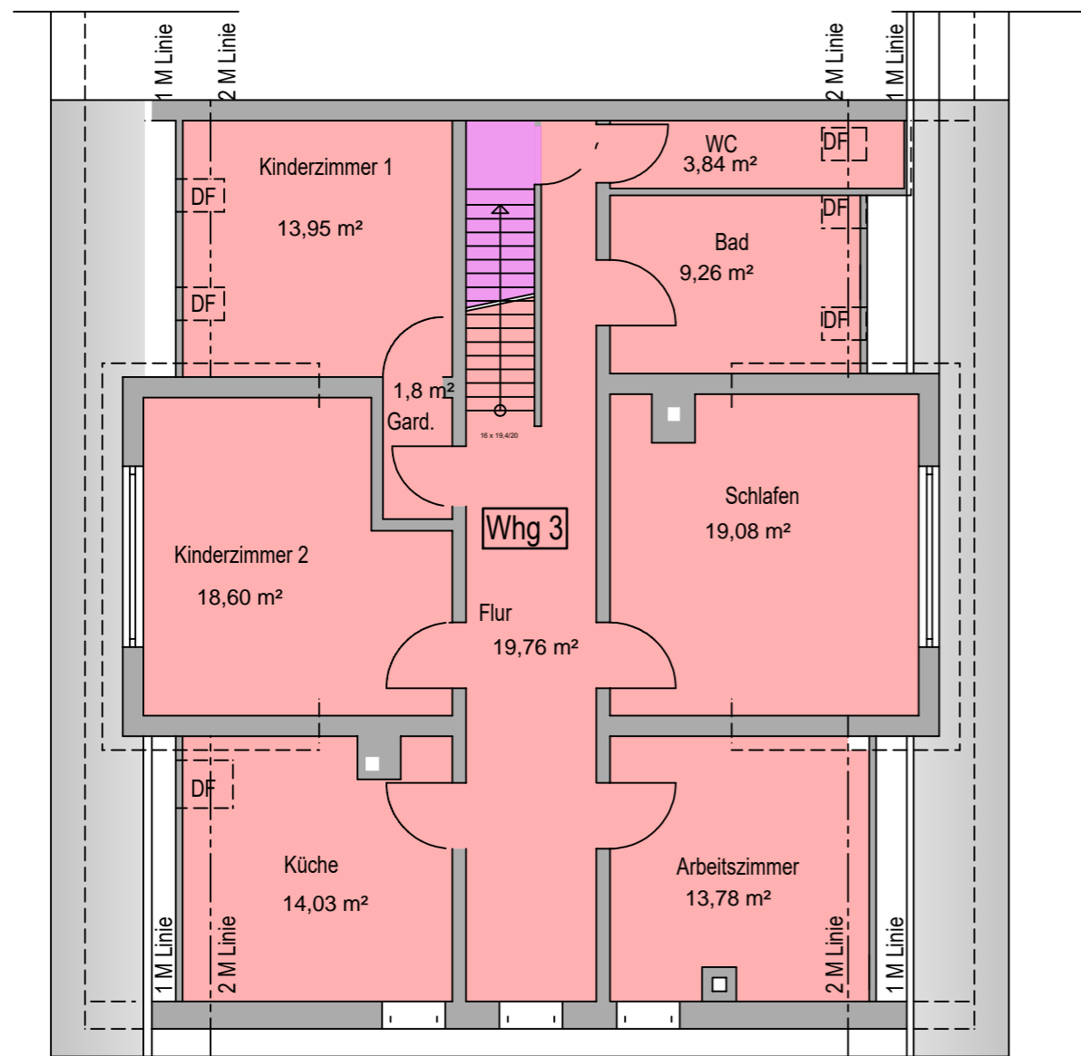
2. Geschoss M.: 1:100
