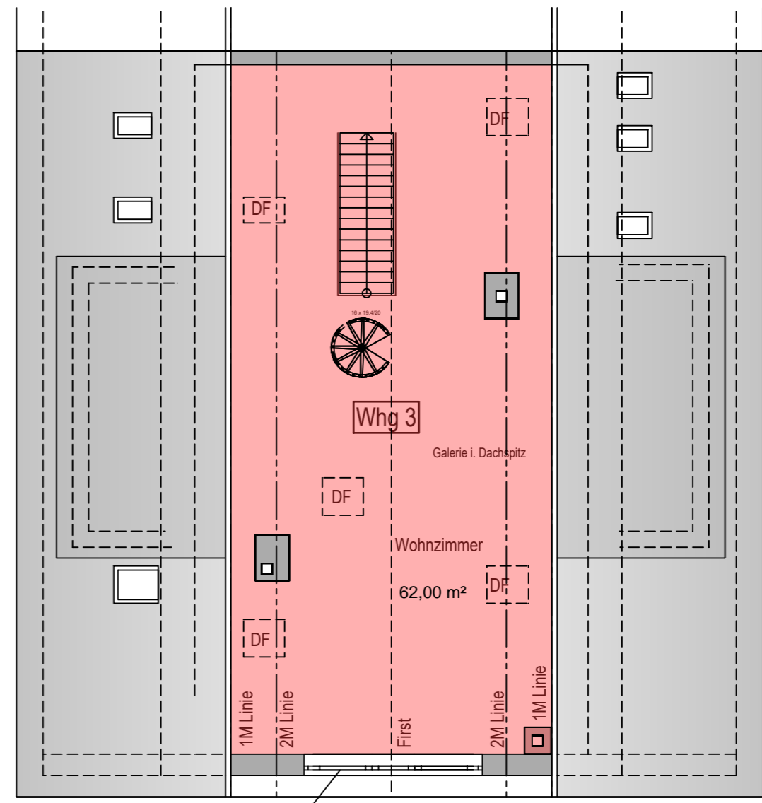
3. Geschoss M.: 1: 100
