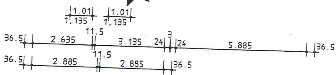
GRUNDRISS DACHGESCHOSS
