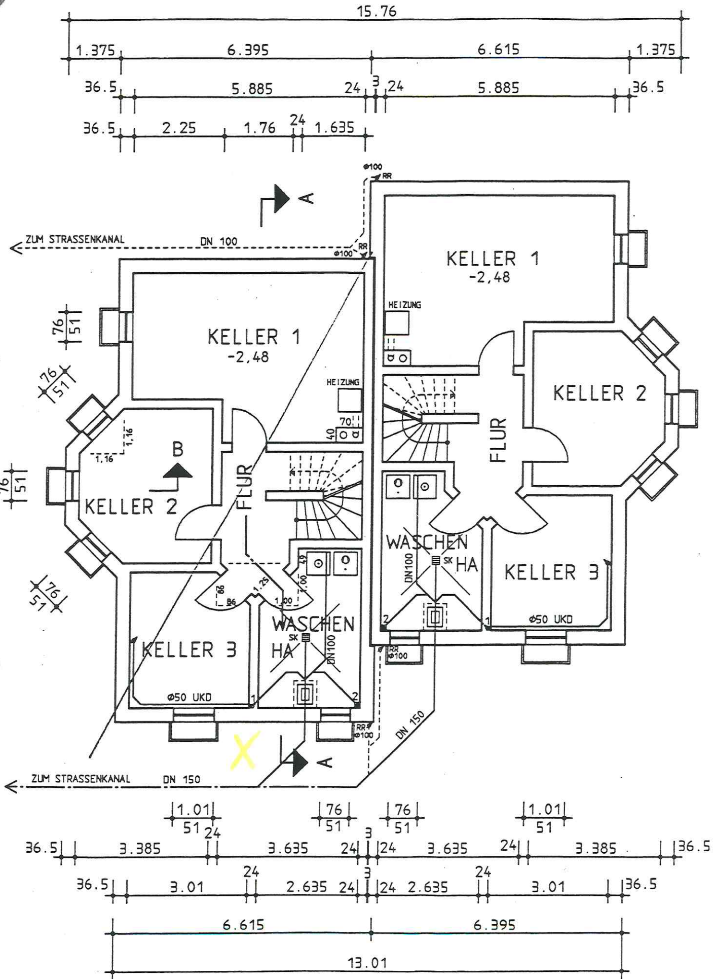
GRUNDRISS KELLERGESCHOSS
