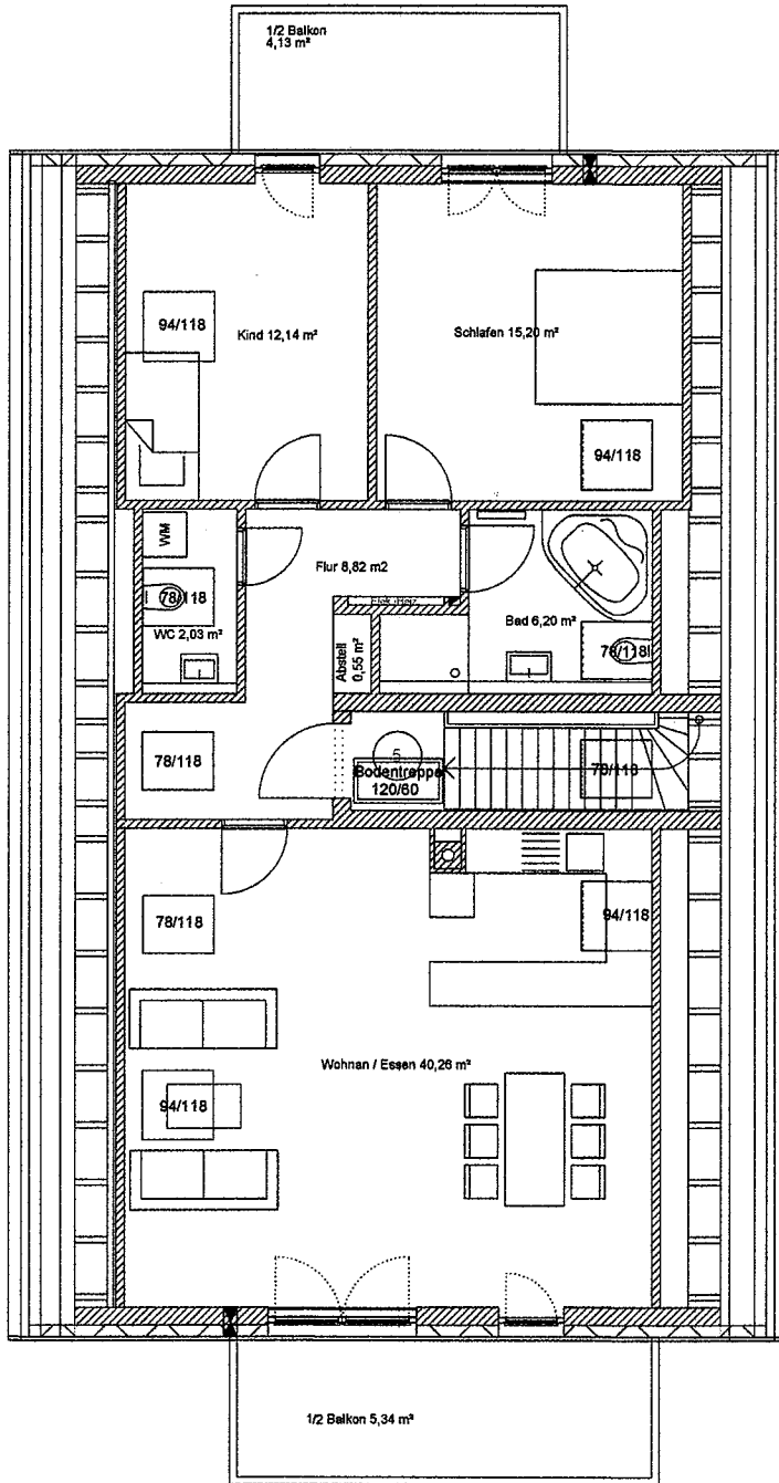
Dachgeschoß
