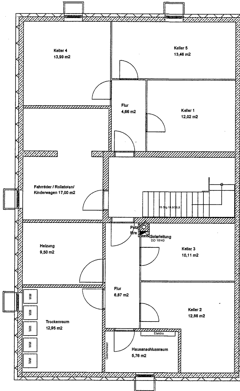
Kellergeschoß
