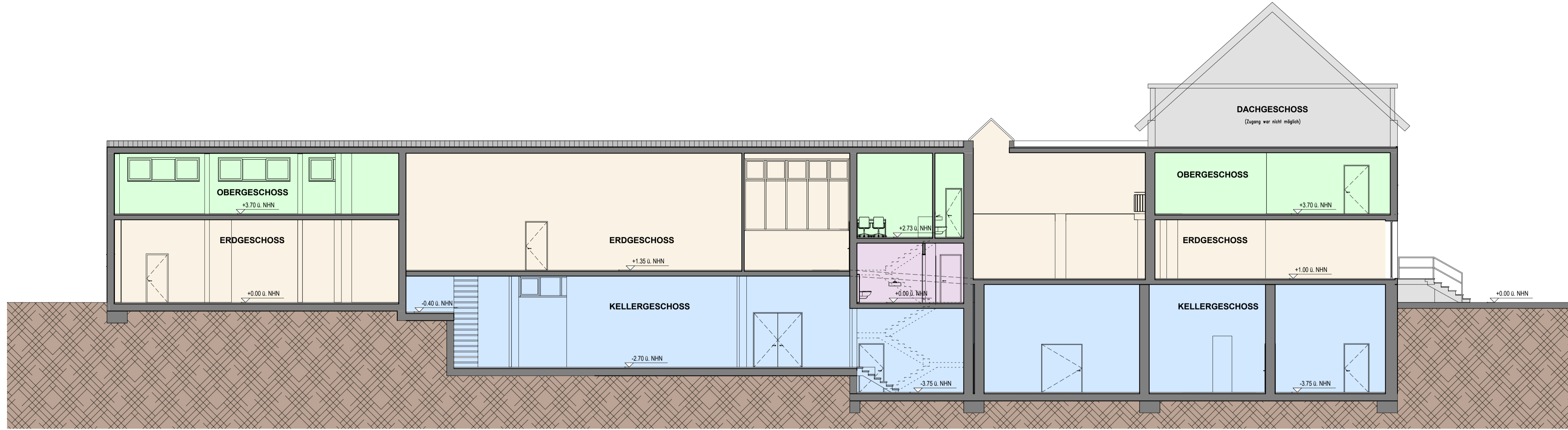
SCHNITT A-A
