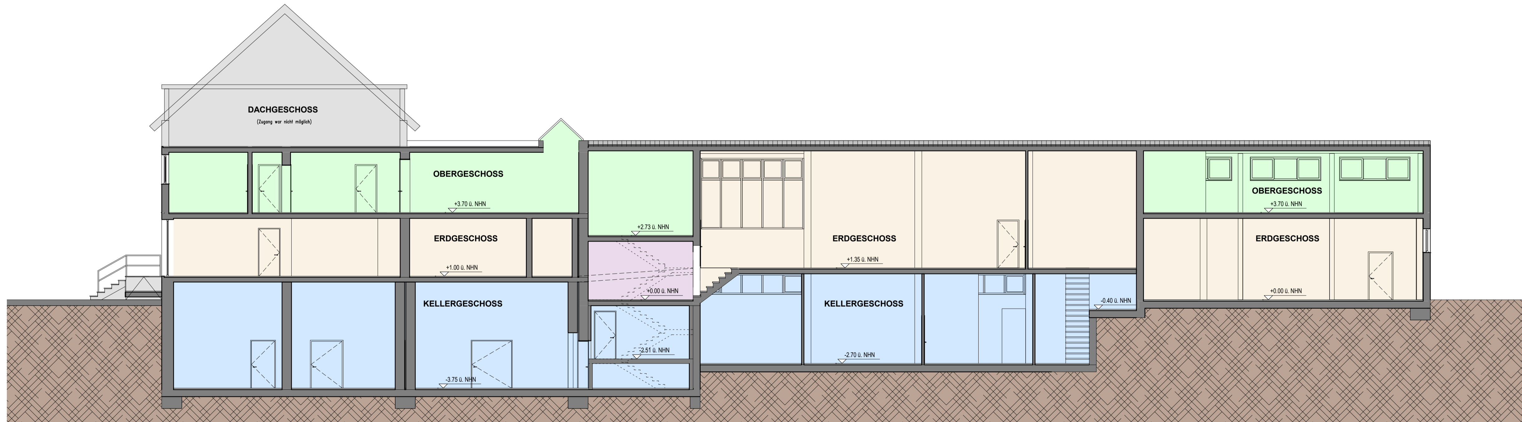
SCHNITT B-B
