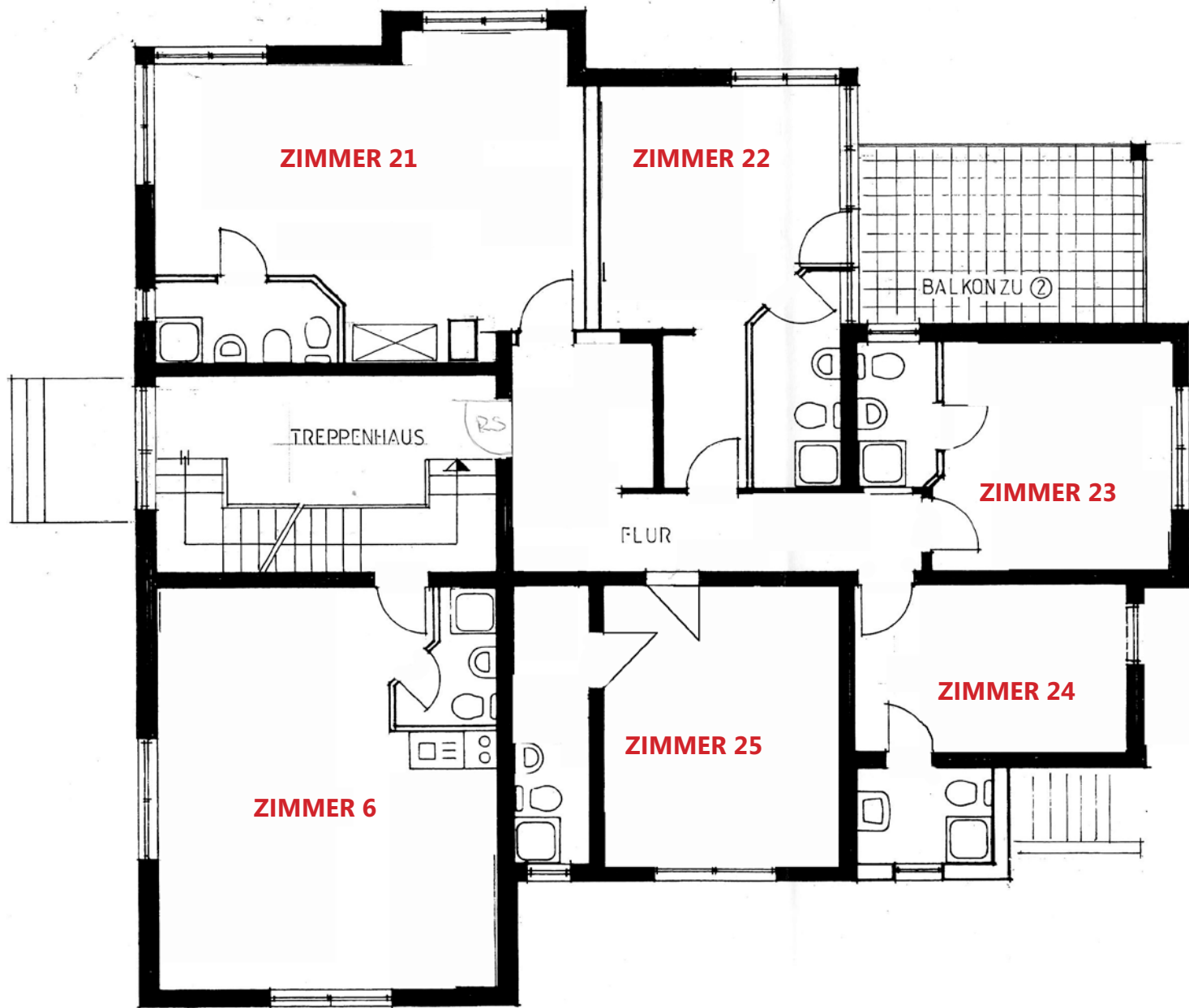
Grundriss OBERGESCHOSS - HOTEL
