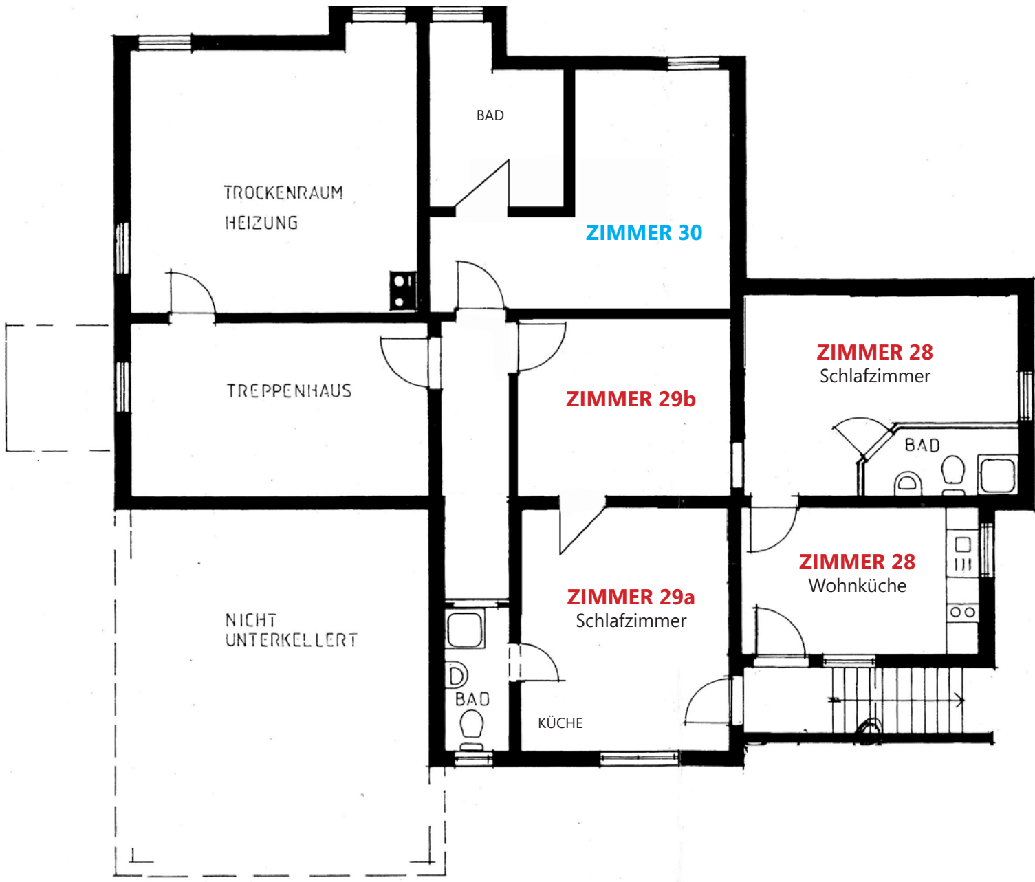
Grundriss UNTERGESCHOSS - HOTEL
