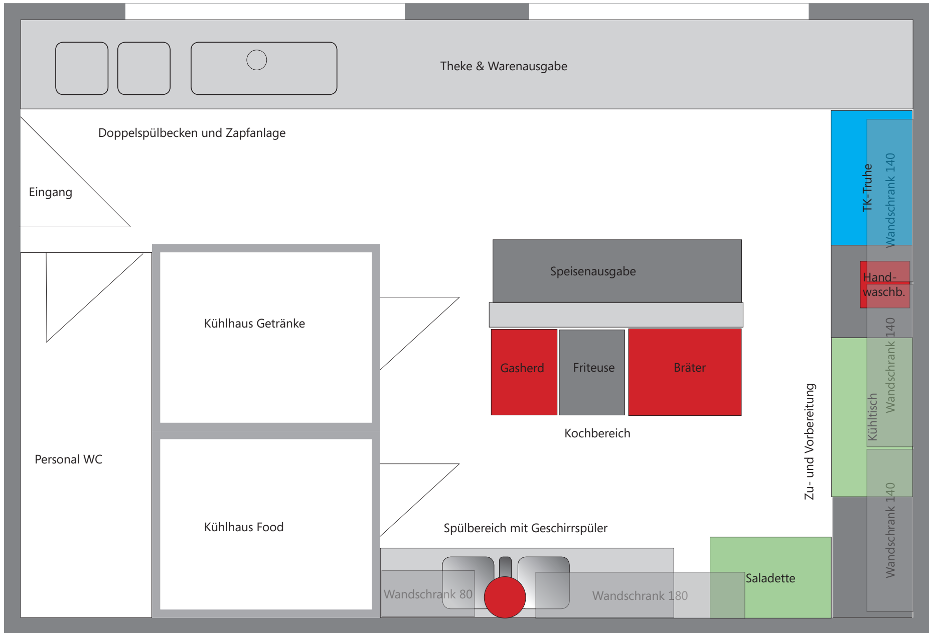
Grundriss Steakhaus mit Gastro-Nutzung
