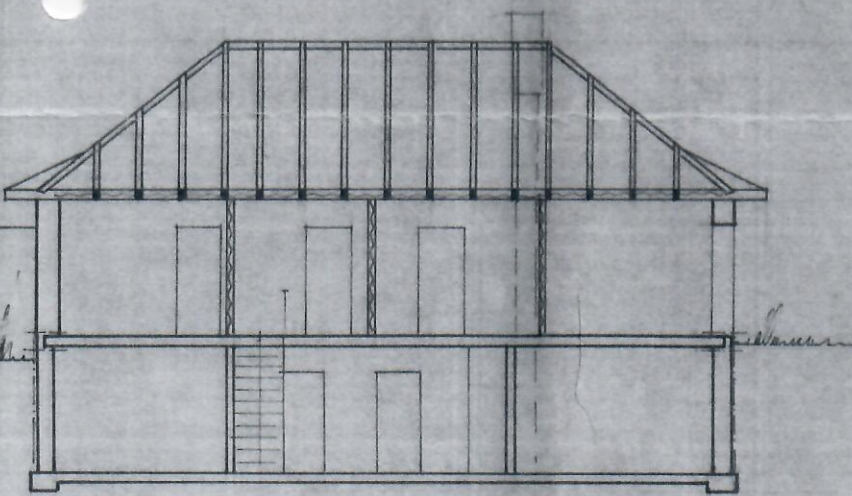
LÄNGSSCHNITT
