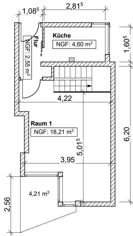
Grundriss OG
