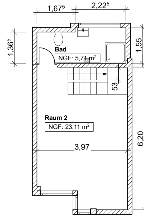
Grundriss UG
