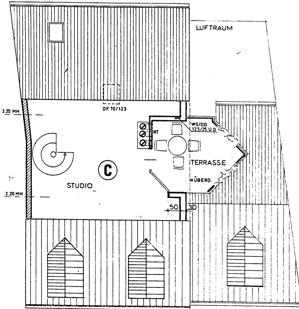
NEUPLANUNG STUDIOGESCHOSS
