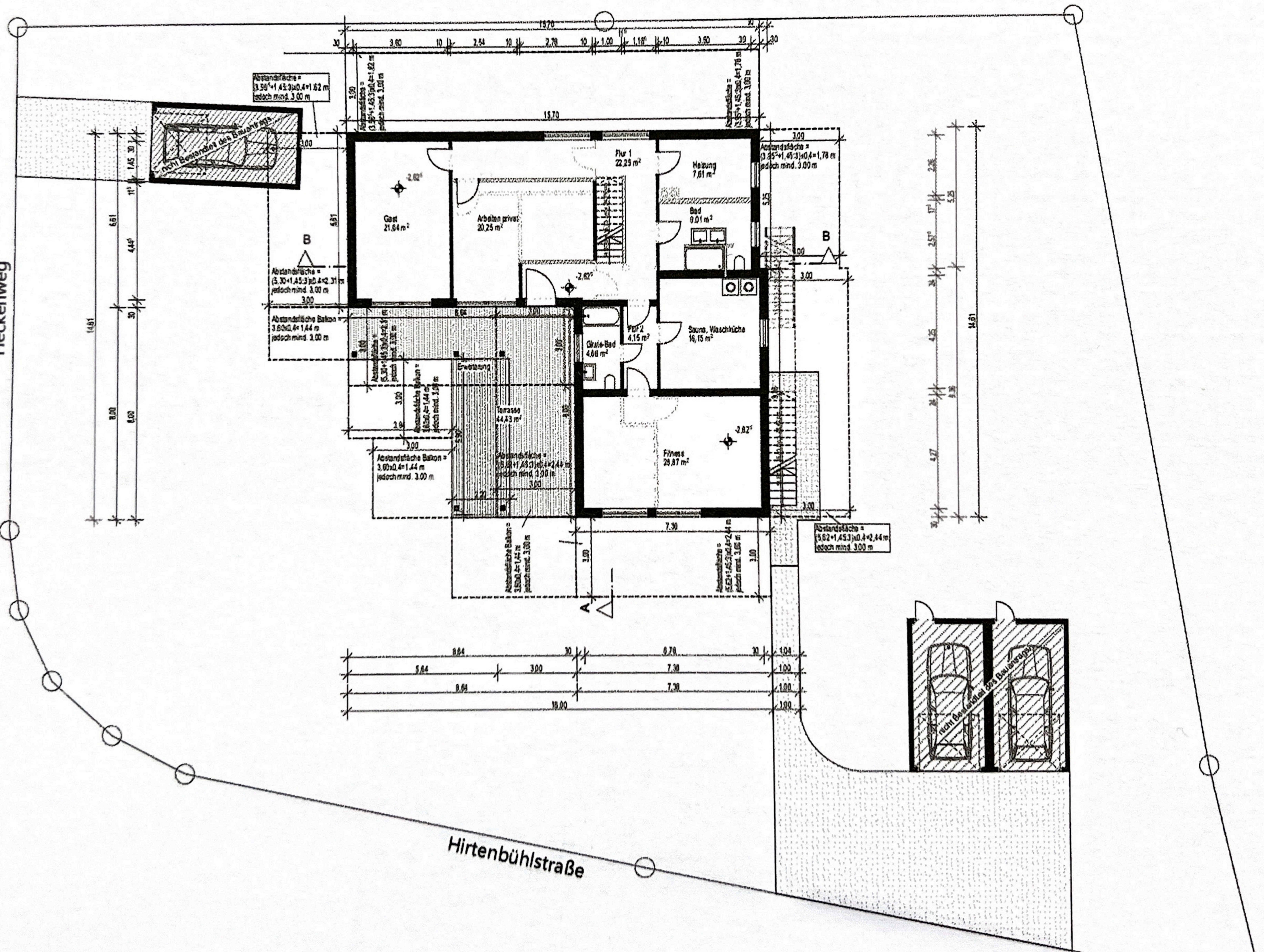
GRUNDRISS KELLERGESCHOSS MIT AUSSENANLAGEN, M 1:100
