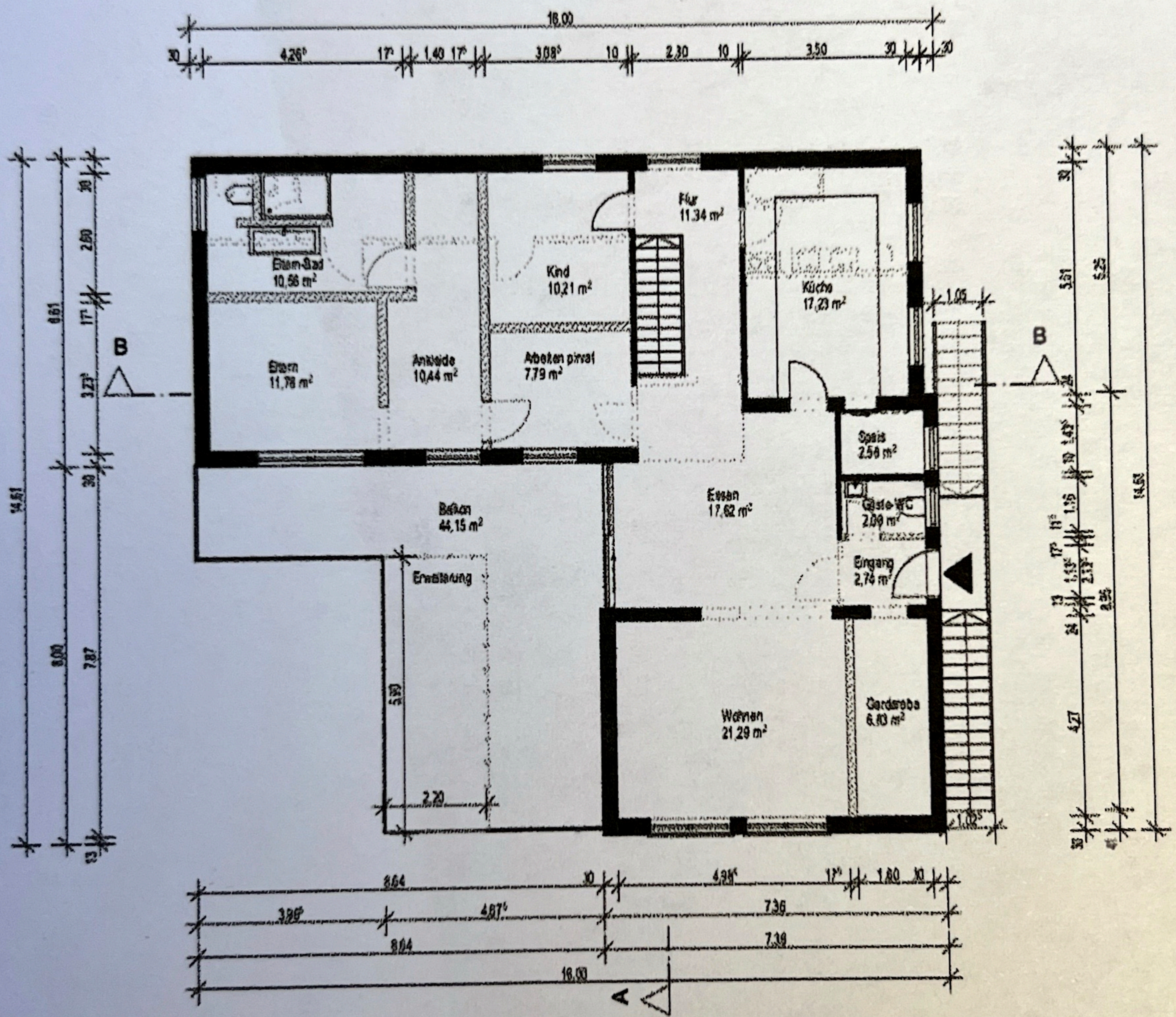
GRUNDRISS ERDGESCHOSS, M 1:100
