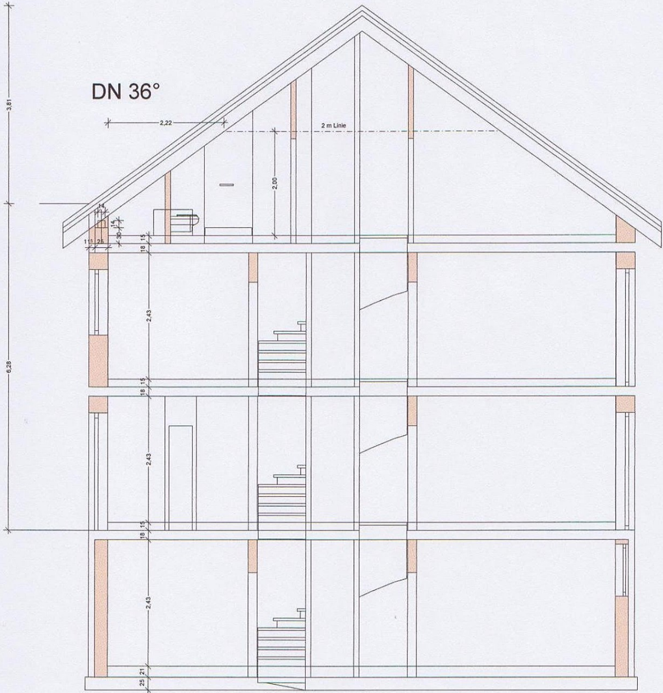
BA 13 Haus 17/18 Schnitt Stand 27.03.2009
