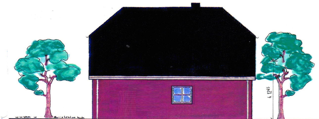
EINFAMILIENHAUS 7.40 x 9.50 m ANSICHT SÜD
