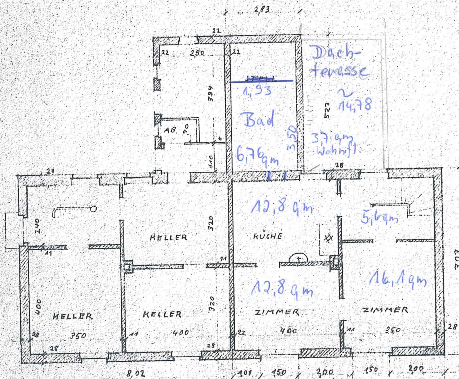
ERD GESCHOSS
