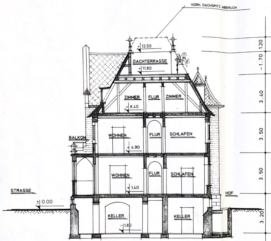
QUERSCHNITT
