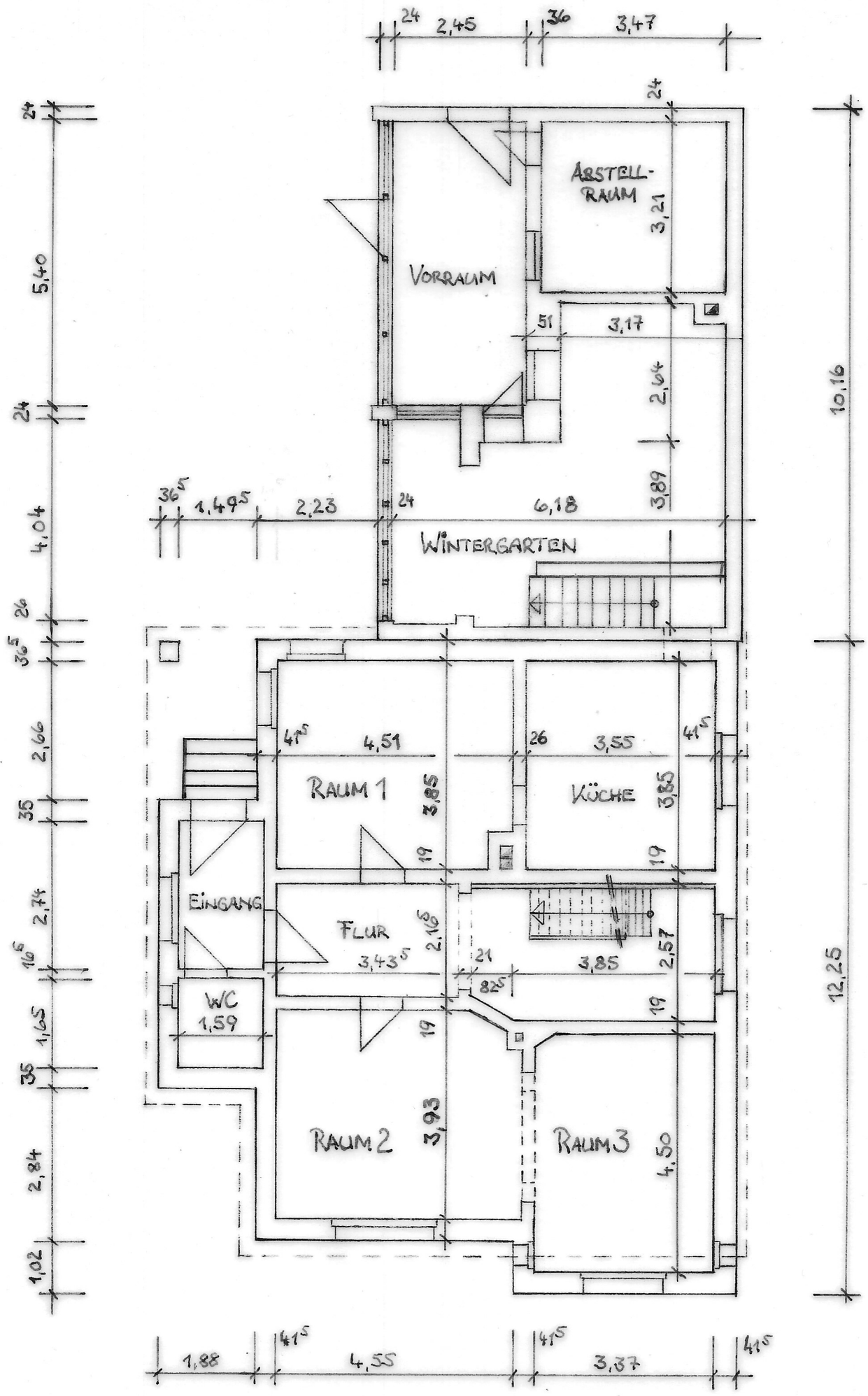
GRUNDRISS EG
